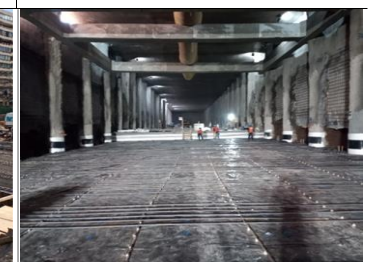
(03.08.2020), Losa Intermedia 63.- (Dm 4.233,5 - 4.263). Se coloca la Armadura de la Losa.
