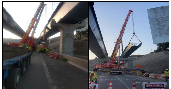
Viaducto El Salto: montaje de vigas tramo 2 ramal C. Empresarial.
